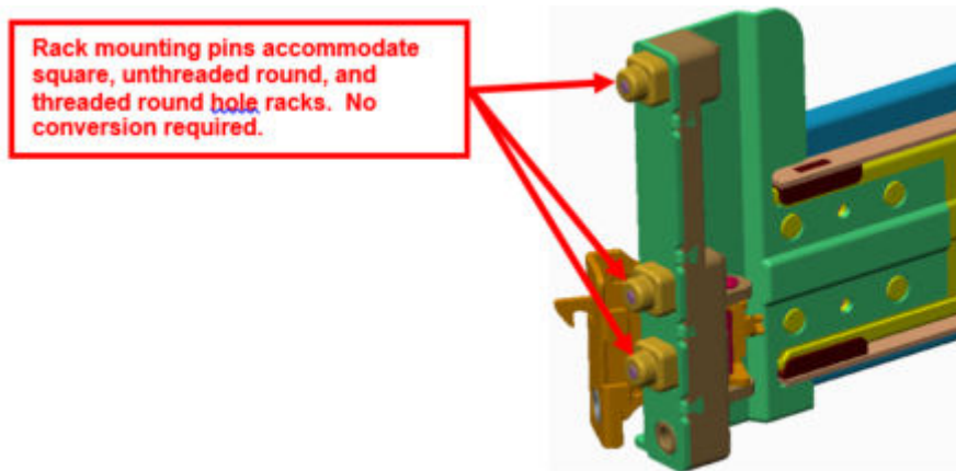
그림 10. 드롭인/스태인 슬라이딩 레일 마운팅 인터페이스
