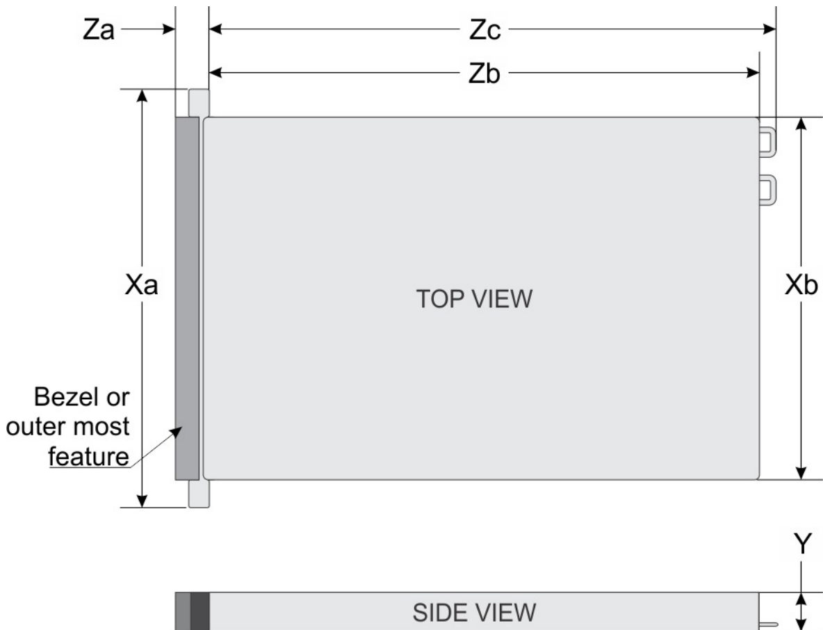
그림 18 . PowerEdge R450 새시 크기
